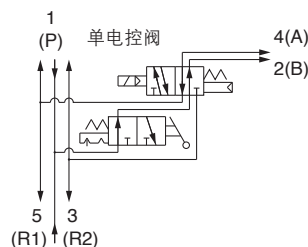
回路图 (安装单电控阀的例)
