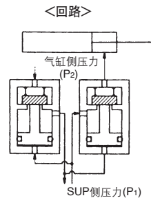
VVQ1000-FPG-02 1组 ※VQ1000-FPG-C6M5-D 2个
