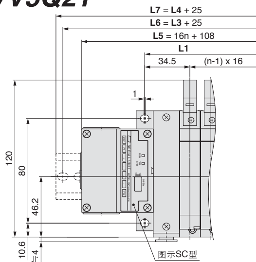
防尘型SI单元
