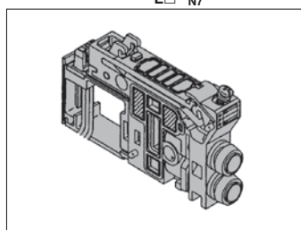
EXH塞板组件 VVQ1000-19A- F□ C3, C4 P□ C6, M5 L□ N1, N3 N7
