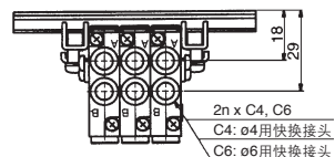
VVQ1000-FPG-02 1组 ※VQ1000-FPG-C6M5-D 2个
