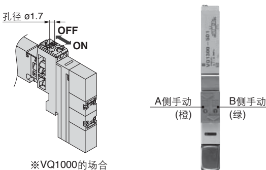
※VQ1000の場合
