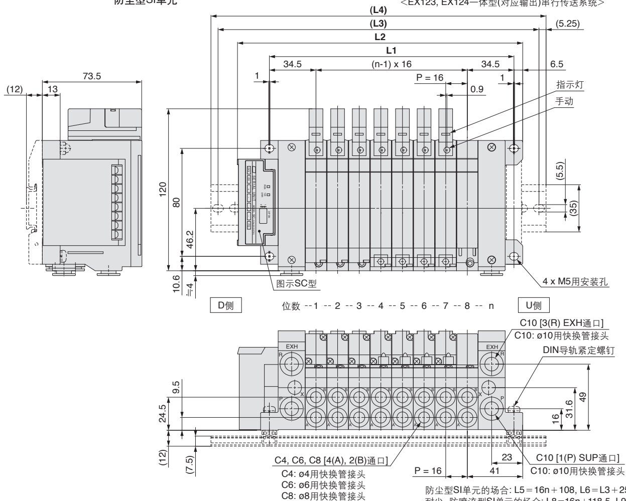
尺寸表
