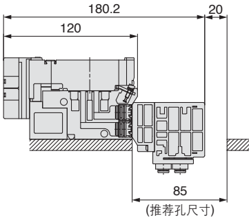
底配管时(VVQ2000-23A-B□)
