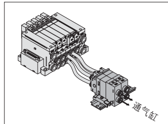
中位止回块(分置型) VVQ2000-FPG-□□-□
