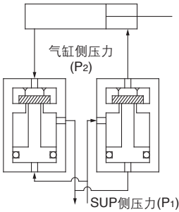
<单向阀动作原理图>
