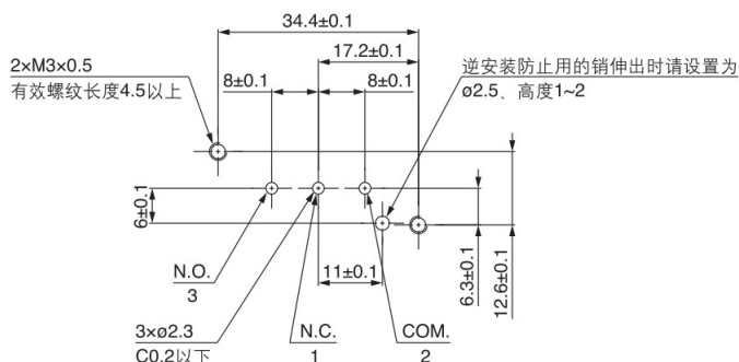
推荐接口尺寸
