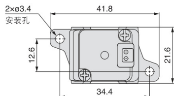
外形尺寸图/底板配管型
